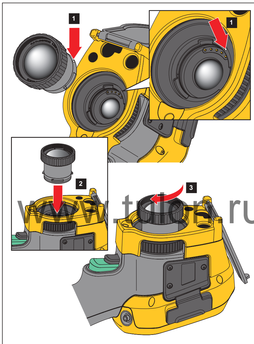
Рисунке 2. Установка дополнительного объектива
